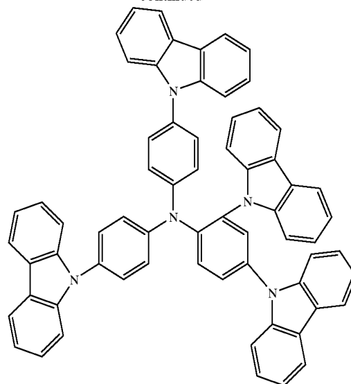
TPA
