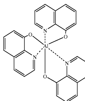
Alq 3
