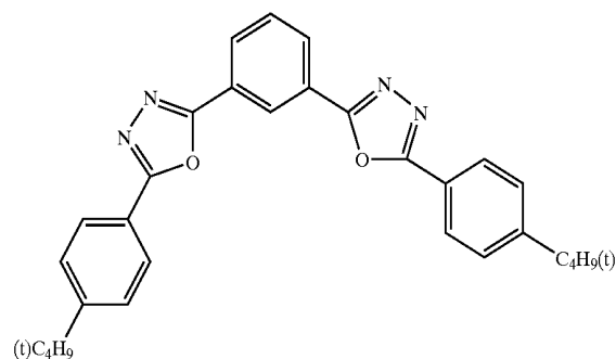
OXD7
